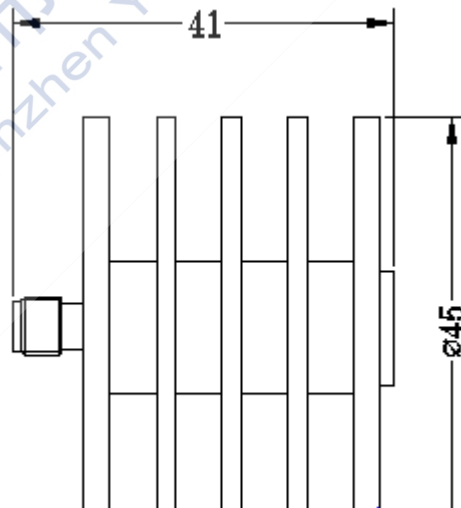
尺寸单位: mm 外形尺寸公差: \pm 2\%
